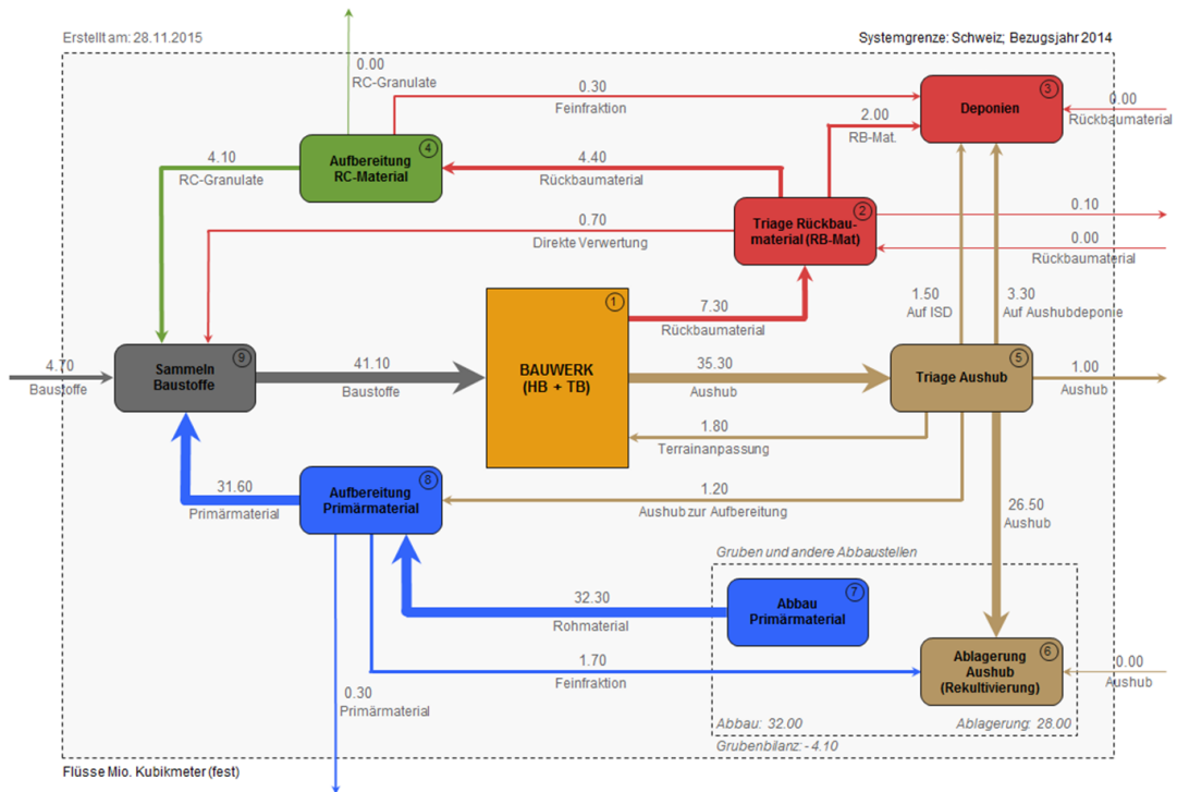
Figur 6 SFA-Diagramm zum Bezugsjahr 2014, Angaben in Mio. Kubikmeter (fest)
