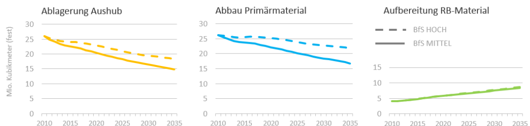
Figur 9 Resultate einiger Materialflüsse der SFA im dynamischen KAR-Modell in Mio. Kubikmeter (fest)
