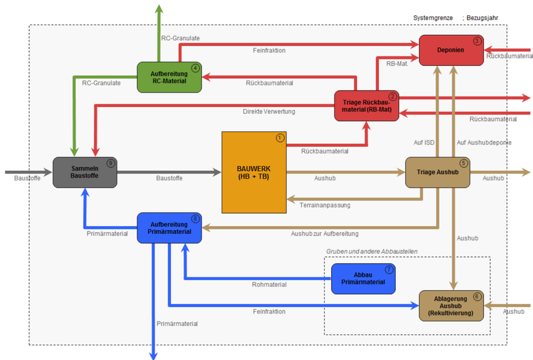
Figur 2 Das Stofffluss-Diagramm für das KAR-Modell, Erläuterungen befinden sich im Text.
