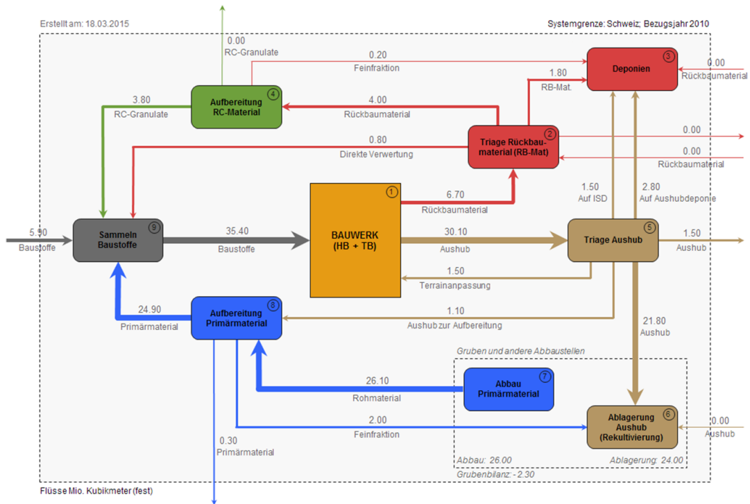
Figur 5 SFA-Diagramm zum Bezugsjahr 2010, Angaben in Mio. Kubikmeter (fest)
