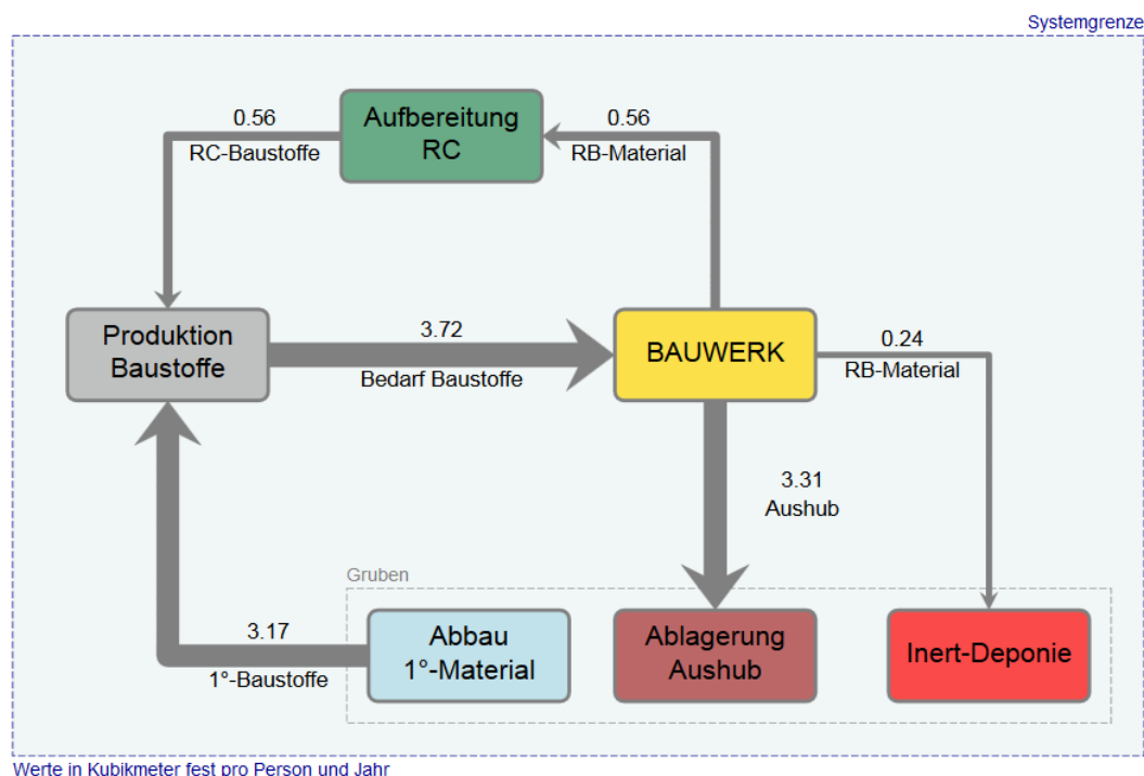
Figur 1 Ein einfaches Modell der mineralischen Materialien. Im Zentrum steht das BAUWERK (Hoch- und Tiefbau), darum die weiteren Prozesse des Systems.
