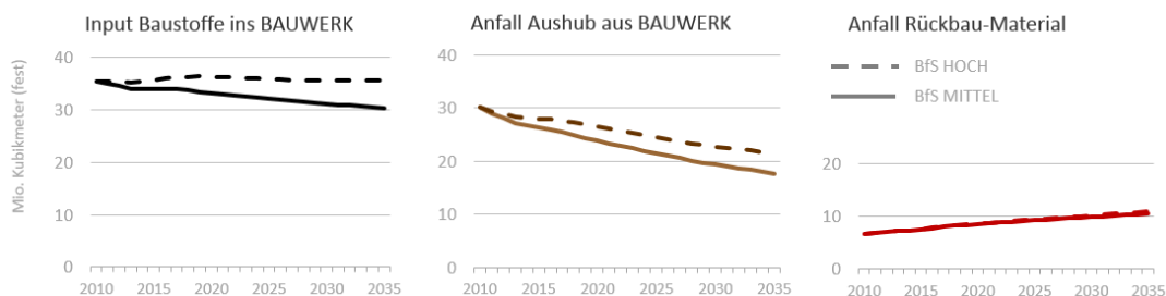
Figur 8 Input- und Outputflüsse des BAUWERK im dynamischen KAR-Modell in Mio. Kubikmeter (fest)
